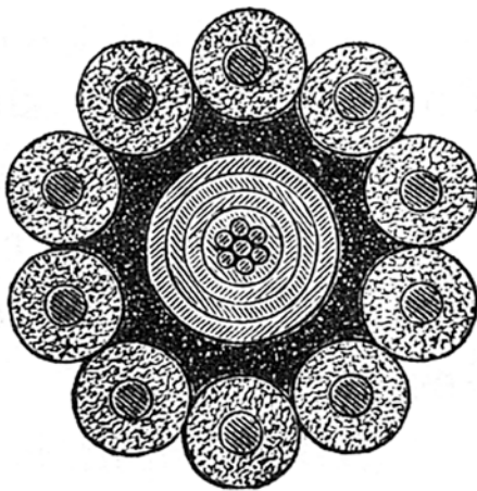
Tiefsee-Kabel vom Jahre 1865.
