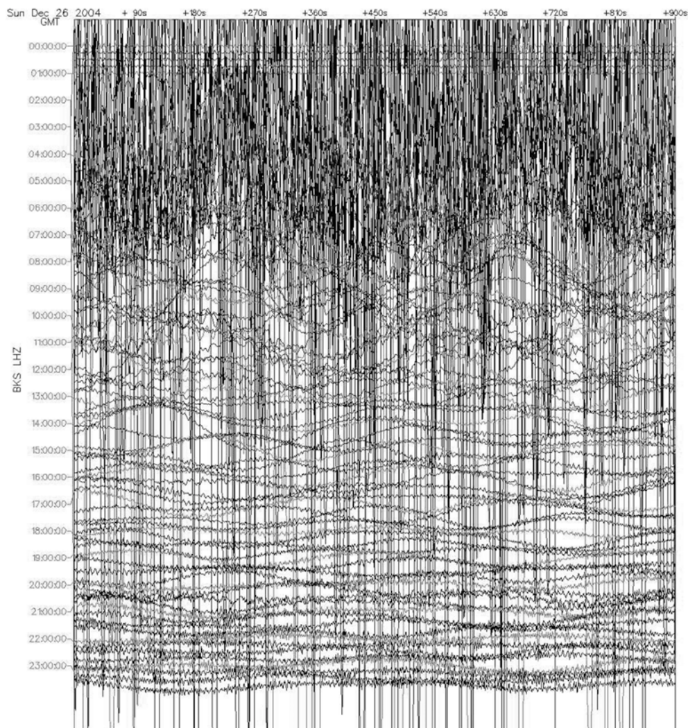
Abb. 1: Seismogramm
